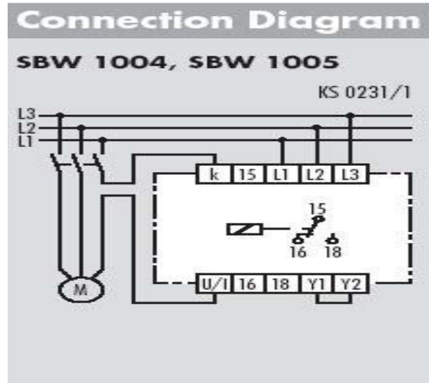
شكل ٩ : مرحل الحماية ضد نقصان الحمل والرسم التخطيطي له.
